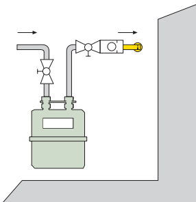
Esempio 2 Sistema tipo “Serie eccesso di flusso”
